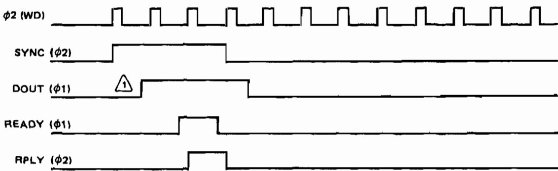
WRITE BYTE (MEMORY OR I/O)
